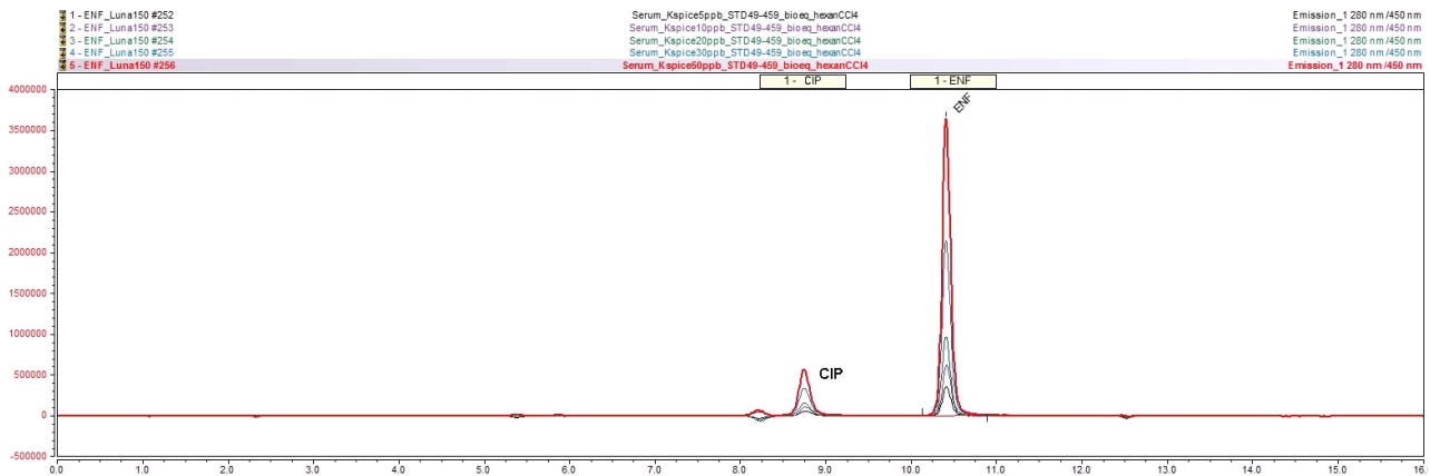
Рис. 2. Хромотограми зразків сироватки крові збагачених різними концентраціями (5, 10, 20, 30, 50 мкг/л) стандартних розчинів енрофлоксацину та ципрофлоксацину.
